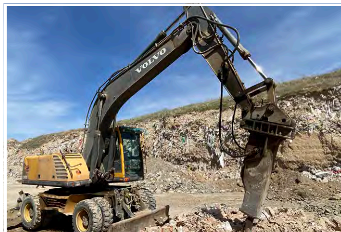
VOLVO EW180B
